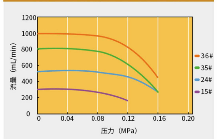
DZ25-6L泵头压力/流量曲线图 (100rpm)
